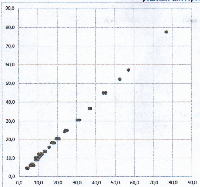
Рис. № 1. Совпадение процентов в таблице 5 диссертации Шпотина В.П. (горизонтальная ось) и таблице 6 диссертации Ларченко Е.В. (вертикальная ось). Каждая точка – пара соответствующих клеток в таблицах.
