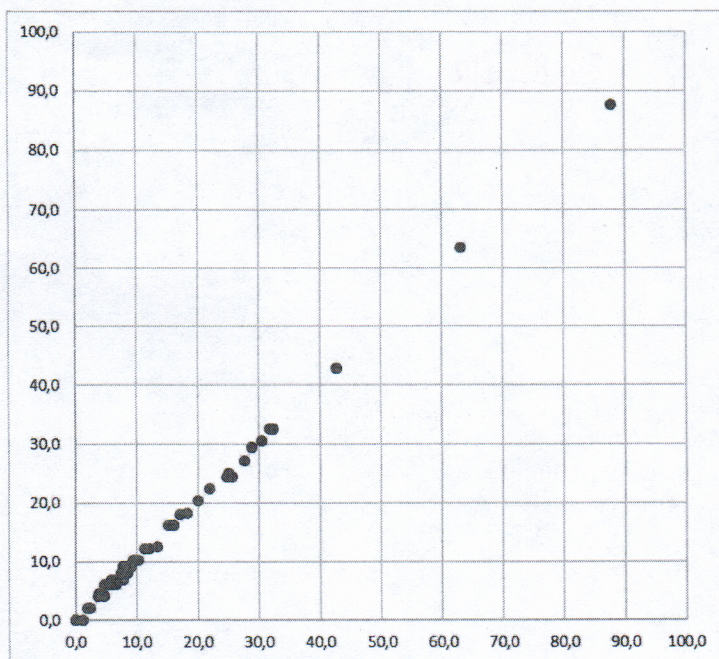
Рис. № 2. Совпадение процентов в таблице 7 диссертации Шпотина В.П. (горизонтальная ось) и таблице 8 диссертации Ларченко Е.В. (вертикальная ось). Каждая точка – пара соответствующих клеток в таблицах.
